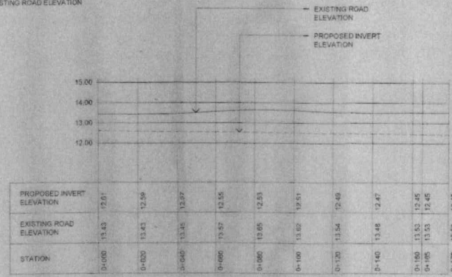
ROAD 2 AMELIA VILLE
